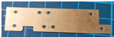
Horní strana šablony, z této strany se vrtá
