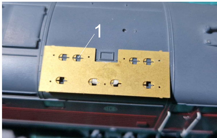
Spodní strana, touto stranou přikládáme šablonu ke střeše, do drážky musí vždy zapadnout vylišovaný profil na střeše modelu
